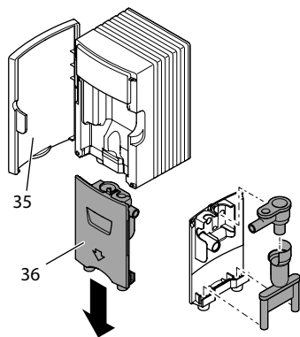
Abb. 17: Milcheinheit ausbauen
