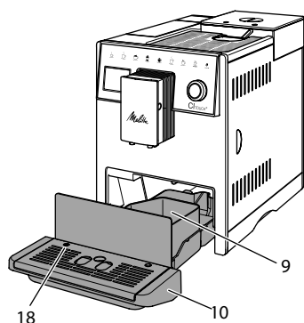
Рис. 10: Поддон для сбора капель, емкость для кофейного жмыха и поплавков
