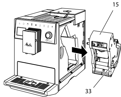
Pav. 14: Plikymo bloko išmontavimas
