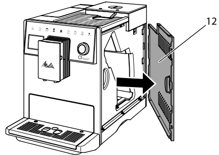
Kuva 13: Sivusuojuksen poistaminen
