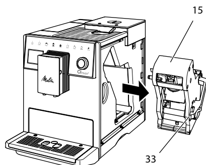
Abb. 14: Brühgruppe ausbauen
