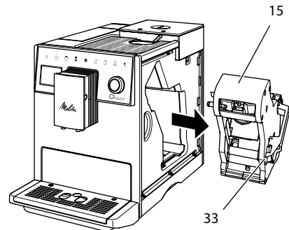
Kuva 14: Suodatusyksikön irrottaminen
