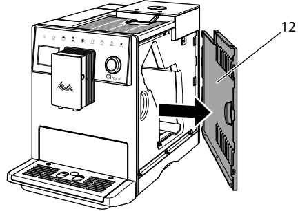
Şek. 13: Yan muhafazanın çıkarılması
