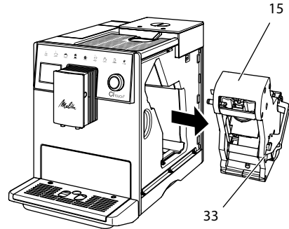
Şek. 14: Demleme ünitesinin çıkarılması
