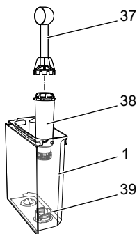
图 16: 安装/拆卸滤水器
