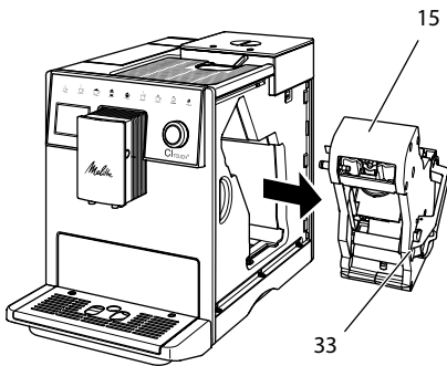
Fig. 14: Demontere kokegruppe
