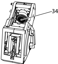
Bild 15: Rengöra bryggenheten
