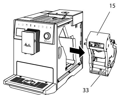
Afb. 14: Zetgroep demonteren
