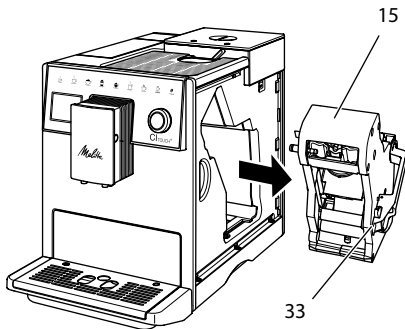
Bild 14: Demontera bryggenheten
